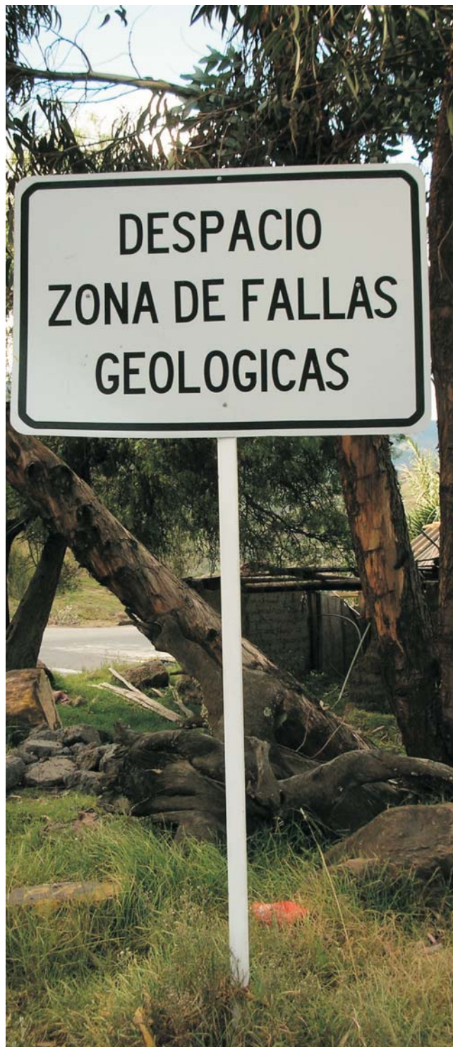
Zona de fallas, de Jose Luis Lopez. GEOFOTOS 2012.
